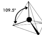
Abb. 2: Tetraedrisches C-Atom
